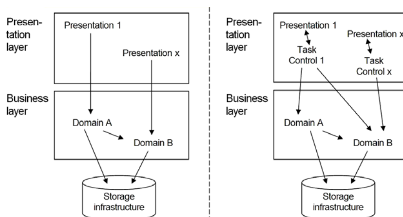
Figuur 2: Twee verschillende lagenmodellen met twee lagen
