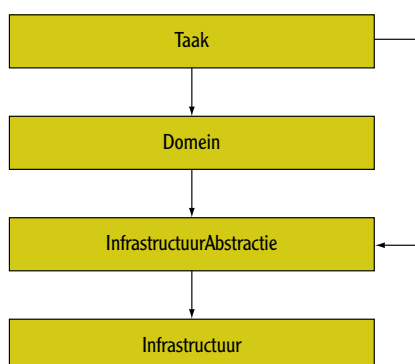
Figuur 1: Een logisch lagenmodel. De Taak-laag bevat de presentatie en taakspecifieke logica en de Domein-laag de domeingenerieke logica conform het 'Logica in Lagen' referentiemodel.
