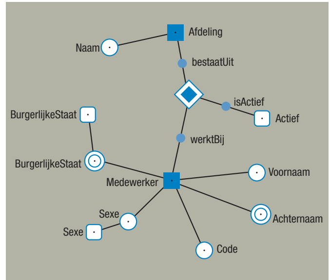
Afbeelding 1: Business keys worden tevens als attribuut gemodelleerd.
